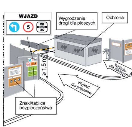
Rys. 1 Organizacja wjazdu do wytwórni mas bitumicznych
