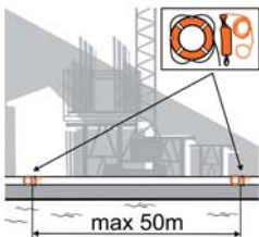
Rys. 1 Koła ratunkowe
