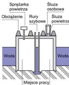
Rys. 4 Praca w kesonach
