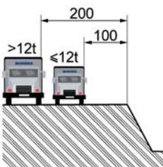
Rys. 12 Minimalne odległości pracy maszyn w sąsiedztwie wykopów
